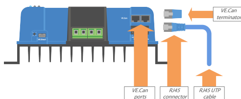
VE.Can-poort, connector, terminator en kabel
